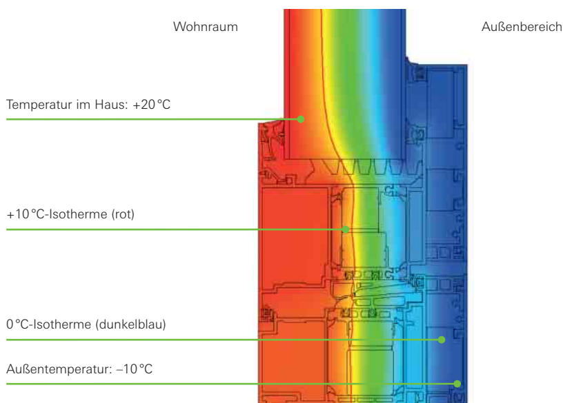
Querschnitt einer hochwärmegeämmten Aluminium Haustür von Schüco. Der Isothermenverlauf zeigt: Trotz der Minusgrade außen herrscht auch direkt an der Haustür eine angenehme Innentemperatur
